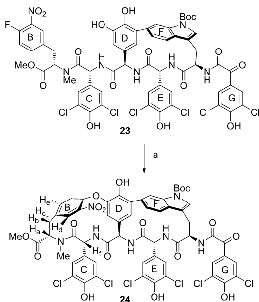
Scheme 3. a) K_2CO_3 , DMSO, 4 Å M.S., 30 °C, 20 h, 60% yield.
